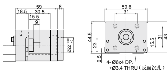
轉接固定座法蘭H1
