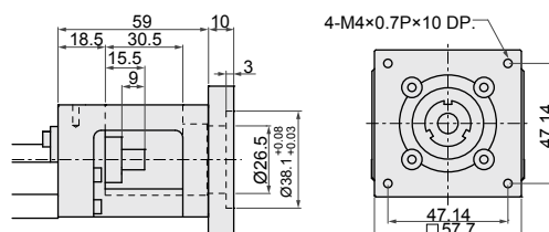
馬達連接法蘭F4
