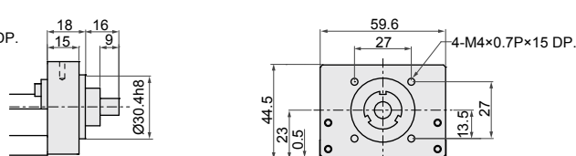
轉接固定座法蘭H1
