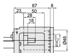
馬達連接法蘭F3
