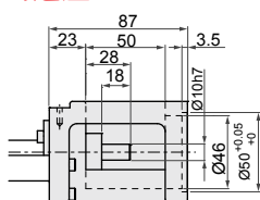
馬達連接法蘭F1
