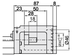
馬達連接法蘭F3
