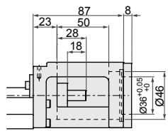
馬達連接法蘭F6
