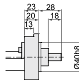
轉接固定座H0
